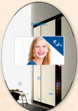
Videocitofono effetto specchio. Monitor da 4,3" a colori con tasti a sfioramento retroilluminati. Videocamera in alluminio a montaggio sporgente con led infrarossi per la visione notturna. Microfono incorporato e suoneria ding dong
